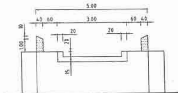
COUPE A-A
